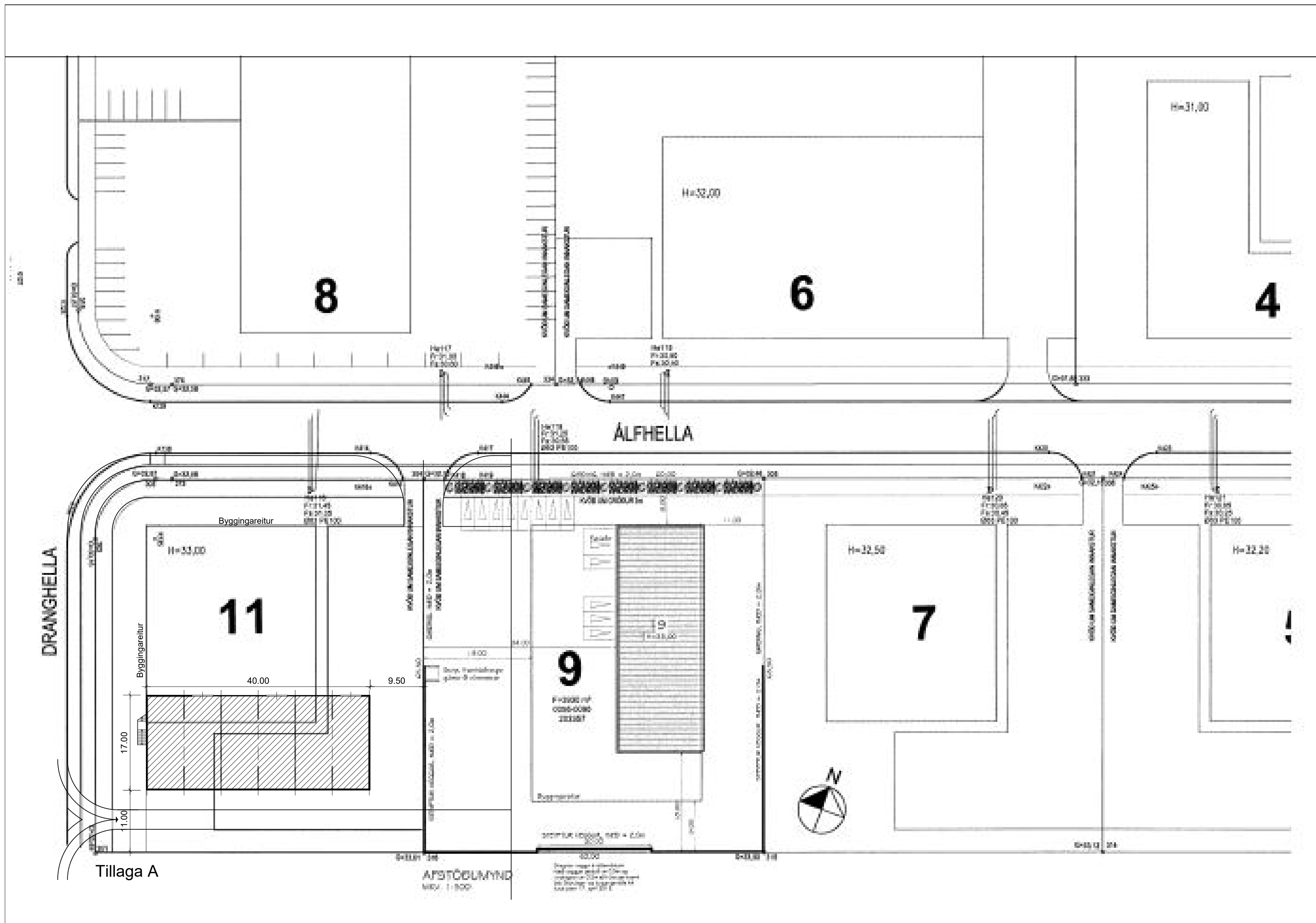
Afstöðumynd 1:500
