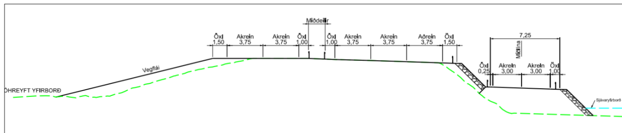
Mynd 4. Þversnið af breikkun Reykjanesbrautar ásamt mögulegum bráðabirgða vegi að Straumi.
