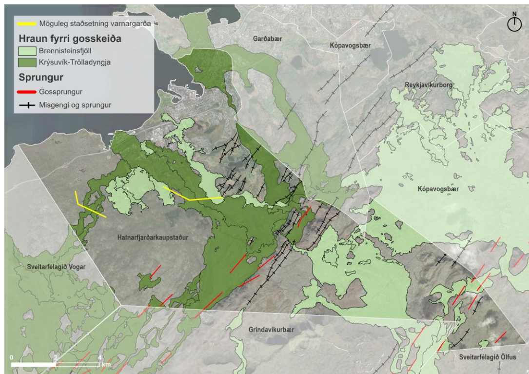
Mynd 3-10. Hraun fyrri gosskeiða og sprungur við byggð í Hafnarfirði. Sýndar eru mögulegar staðsetningar varnargarða.
