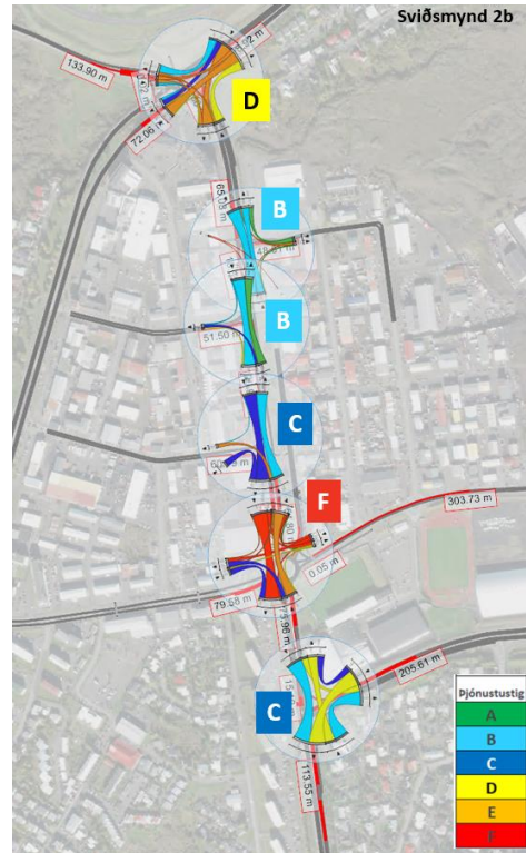
MYND 35 Þjónustustig umferðarstrauma og gatnamóta, ásamt meðalröðum á hámarksklukkustund síðdegis fyrir sviðsmynd 2
