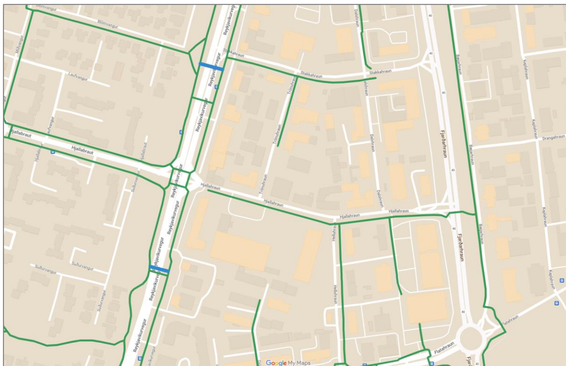
MYND 20 Ákjósanlegar staðsetningar á mislægum göngutengingum sýndar með bláum lit. Við Reykjavíkuregur 56 og Reykjavíkuregur 70.
