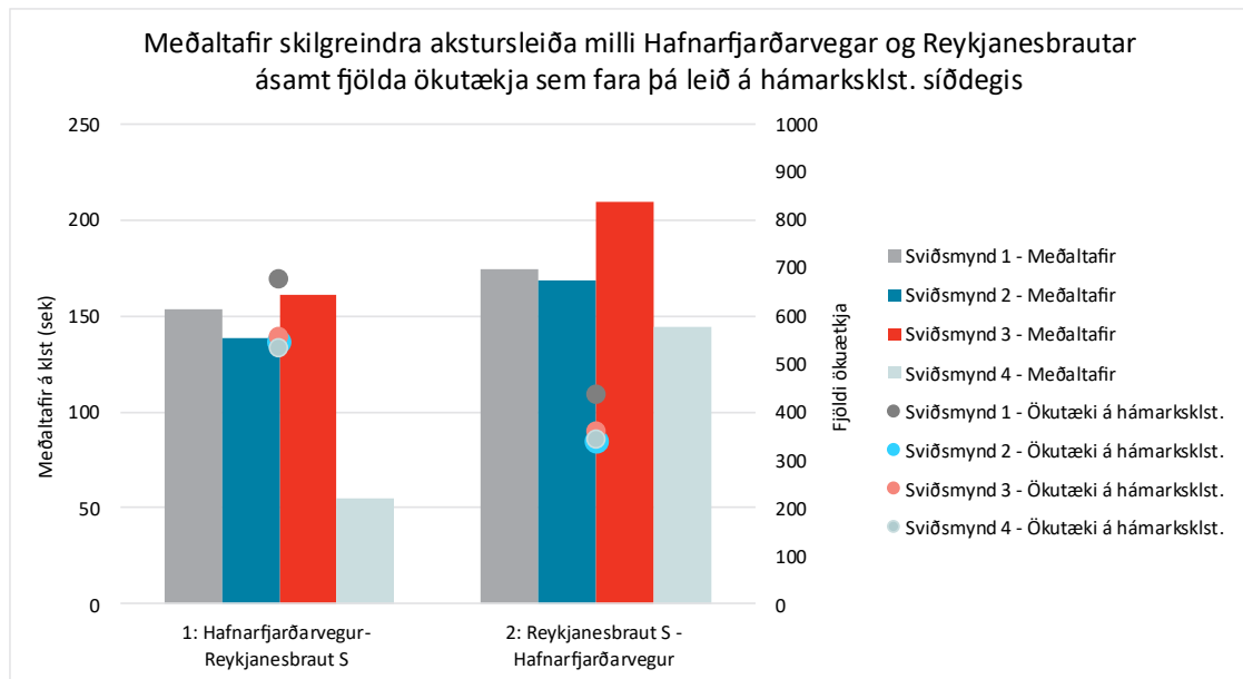
MYND 40 Meðaltafir fyrir akstursleiðir um Fjarðarhraun (1,6 km), milli Hafnarfjarðarvegur og Reykjanesbrautar, á hámarksklukkustund síðdegis (súlur). Fjöldi ökutækja á tilteknum akstursleiðum er sýnt með punktum. Sýndar eru niðurstöður fyrir fjórar sviðsmyndir árið 2040
