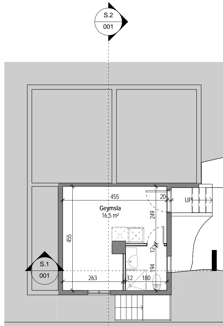
Kjallari 1 : 100
