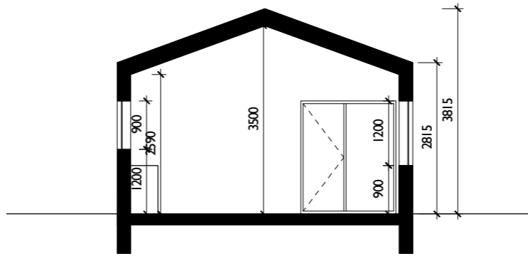
Sneiðing A-A 1:100
