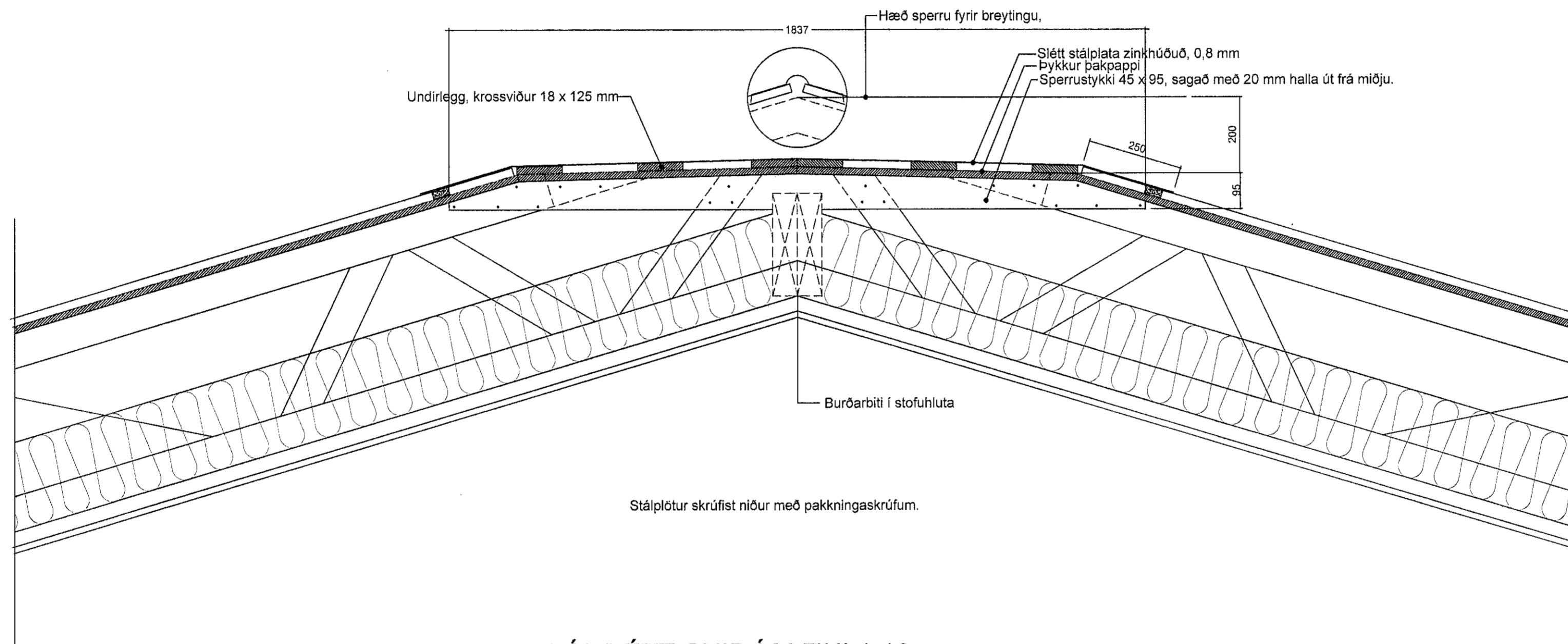
LÓÐRÉTT SNIÐ Í MÆNI 1:10
