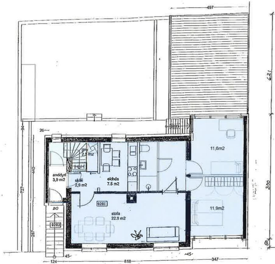
1:100 Grunnmynd 2. hæðar Grunnmynd, 2. hæð
