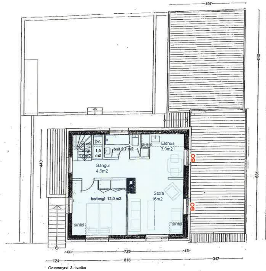
1:100 Grunnmynd 3. hæðar Grunnmynd, 3. hæð
