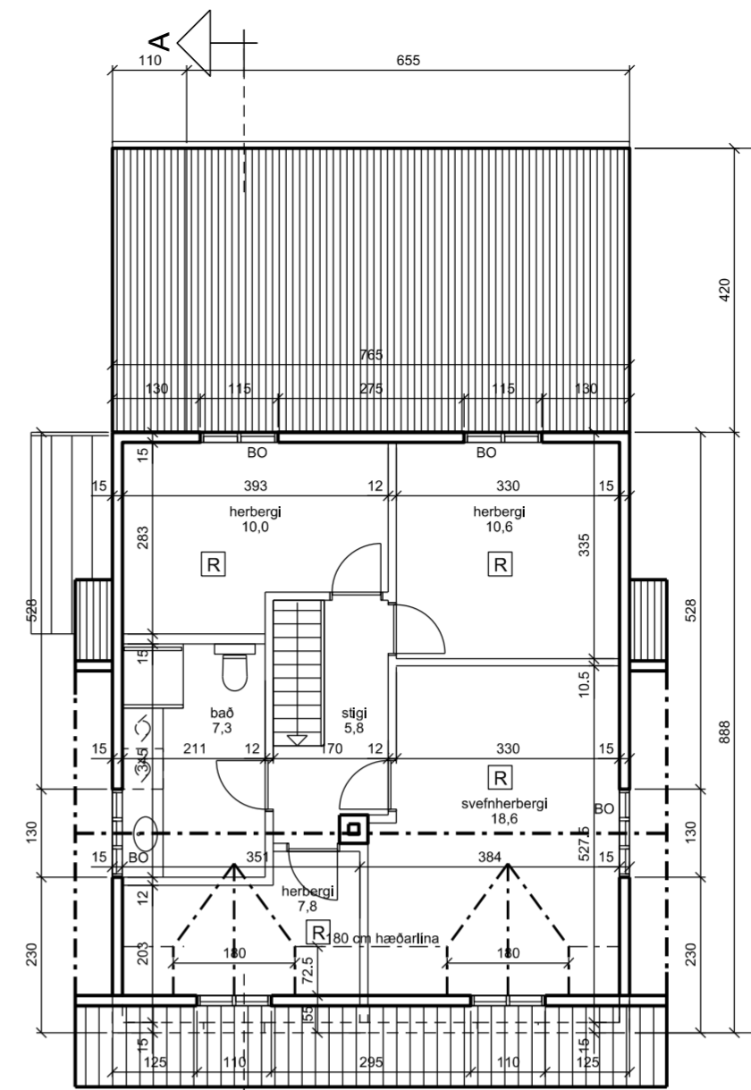
GRUNNMÝND ÞAKHÆÐAR
