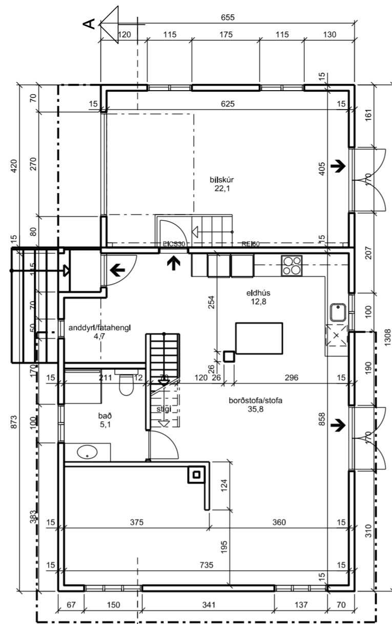
GRUNNMÝND HÆÐAR
