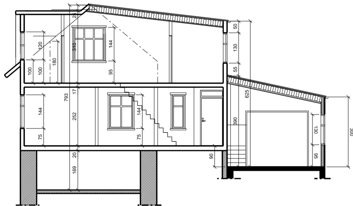
SNEIDING A-A
