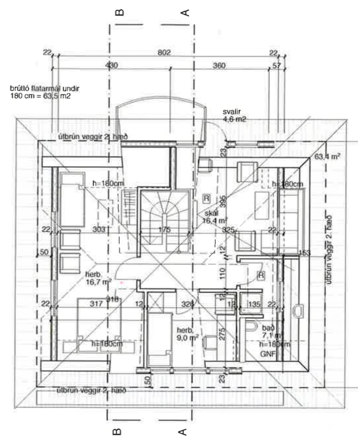
3. Ris 1:100
