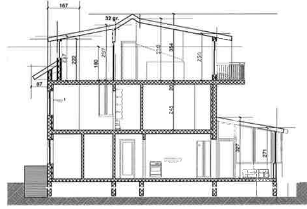
A Skurdmynd 1:100
