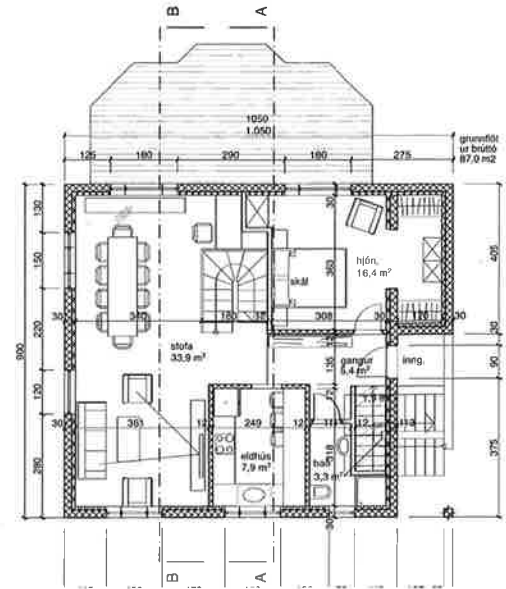
2. 2. hæð 1:100
