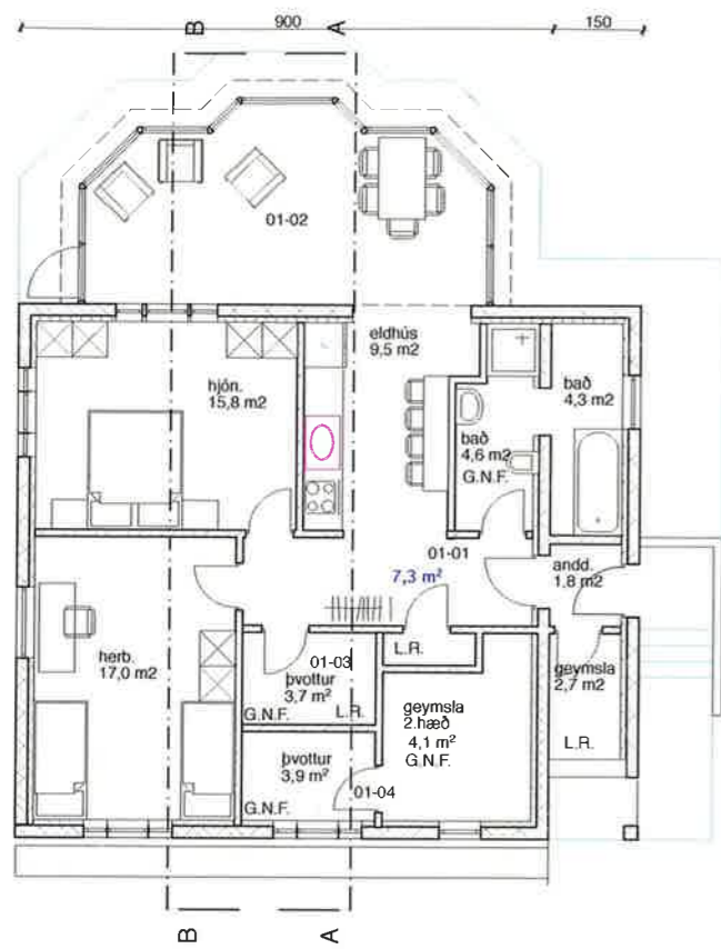
1. Jardhæd 1:100
