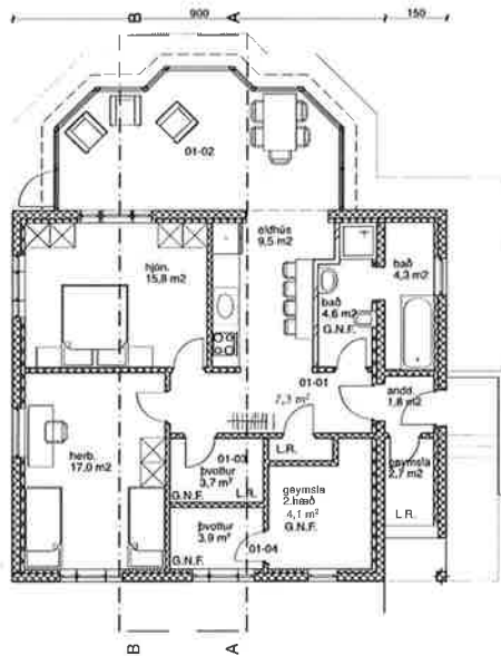
1. Jardhæð 1:100
