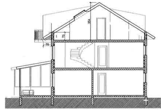
B Skurdmynd 1:100
