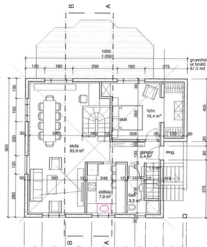
2. 2. hæd 1:100
