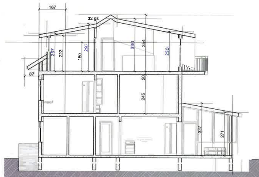
A Skurdmynd 1:100
