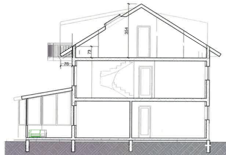
B Skurdmynd 1:100
