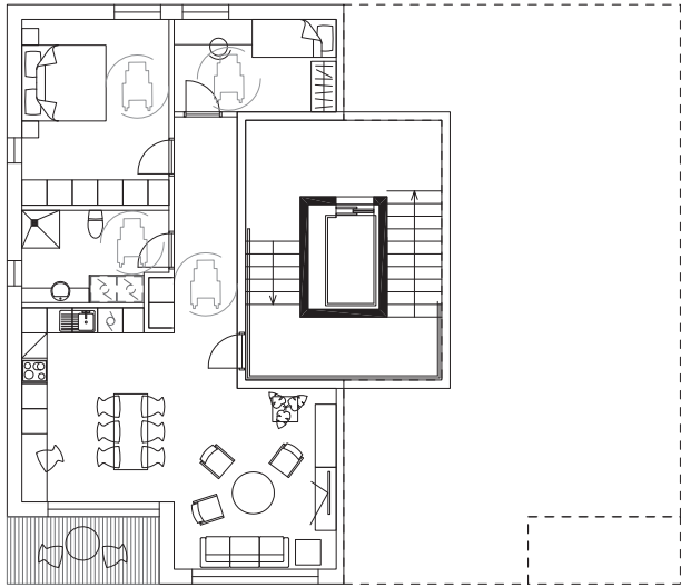
Dæmi um 90 m 2 íbúð
