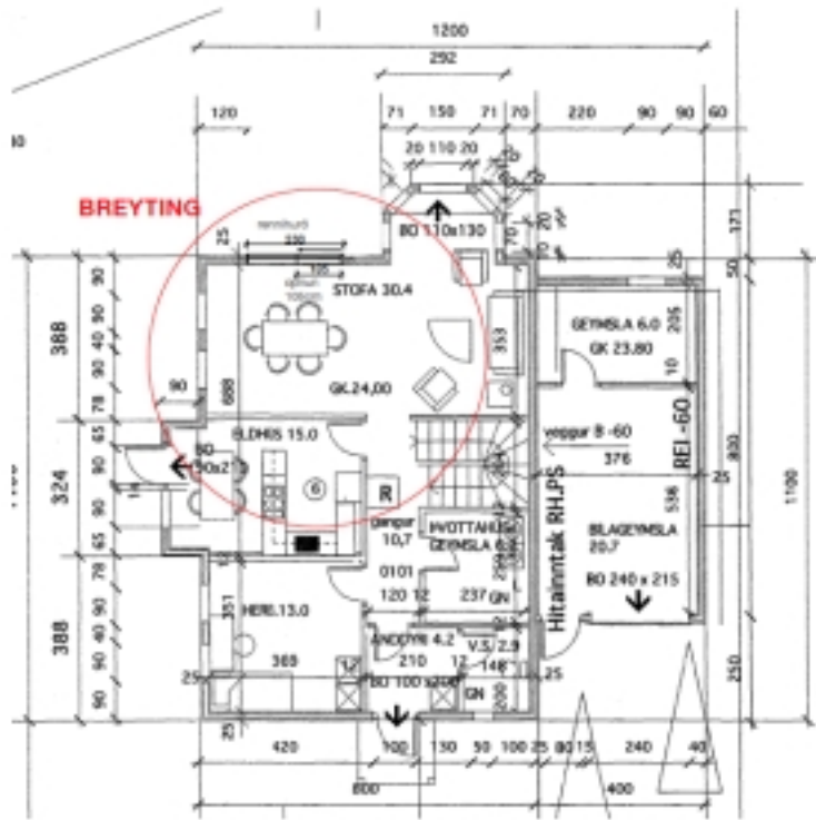
0. GRUNNMYND 1:100
