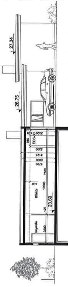
Sníð C - norður 1:100
