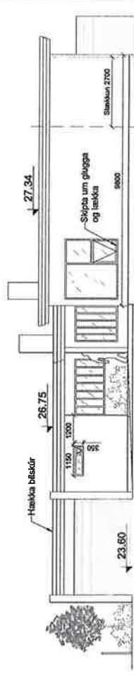
Útlit vestur 1:100
