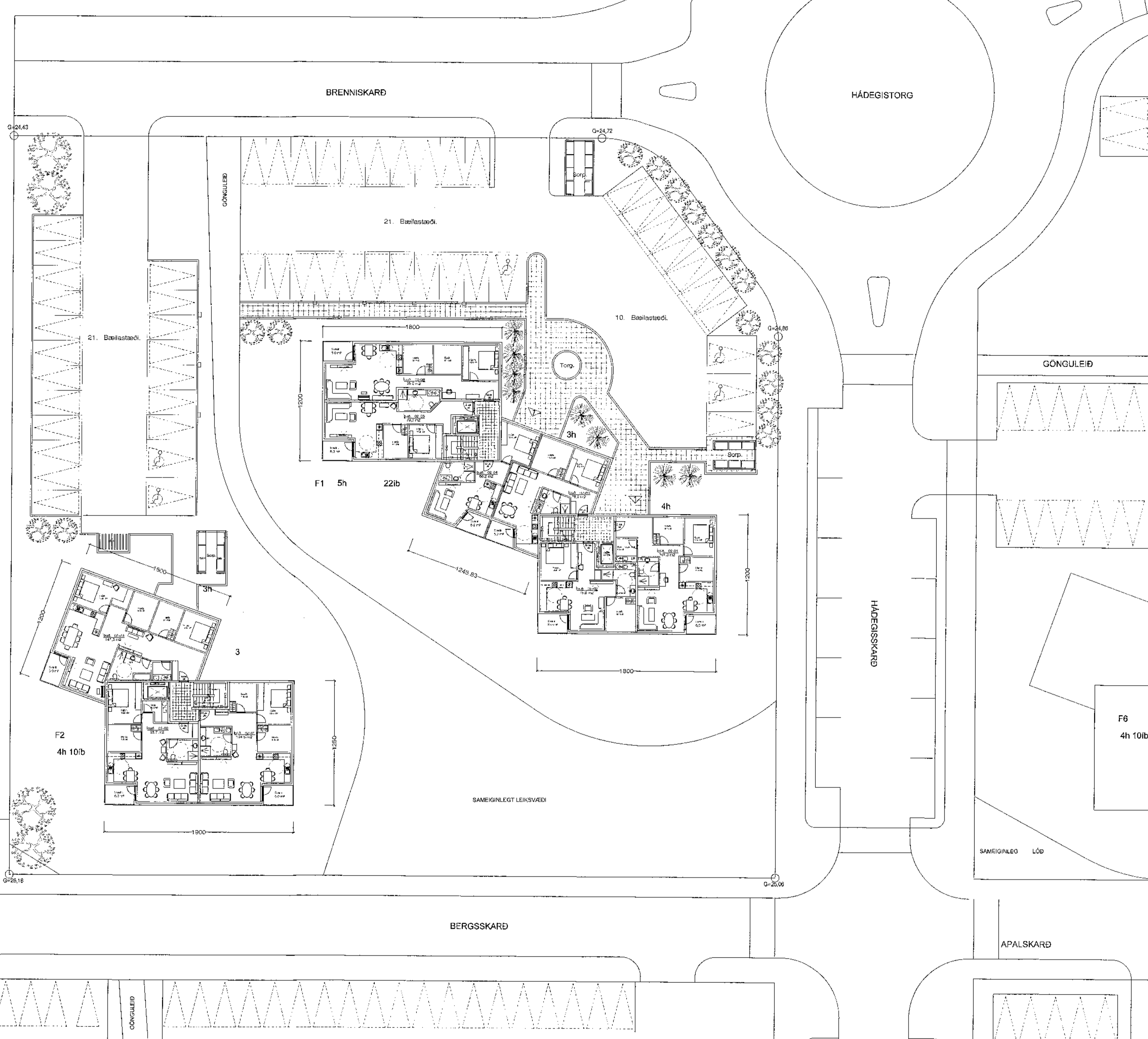
Grunnmynd 2. - 5. hæð. 1 : 200 Stærð. 2. - 3. hæðar. 906,0 m 2
