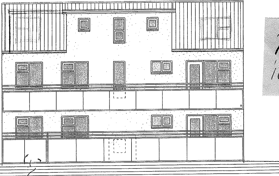
ÚTLIT NORÐAUSTUR MKV. 1:100.
