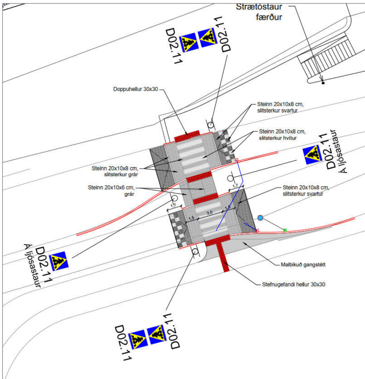
MYND 10 Hellulögð, upphækkuð gangbraut með miðeyju ásamt leiðarlínum.
