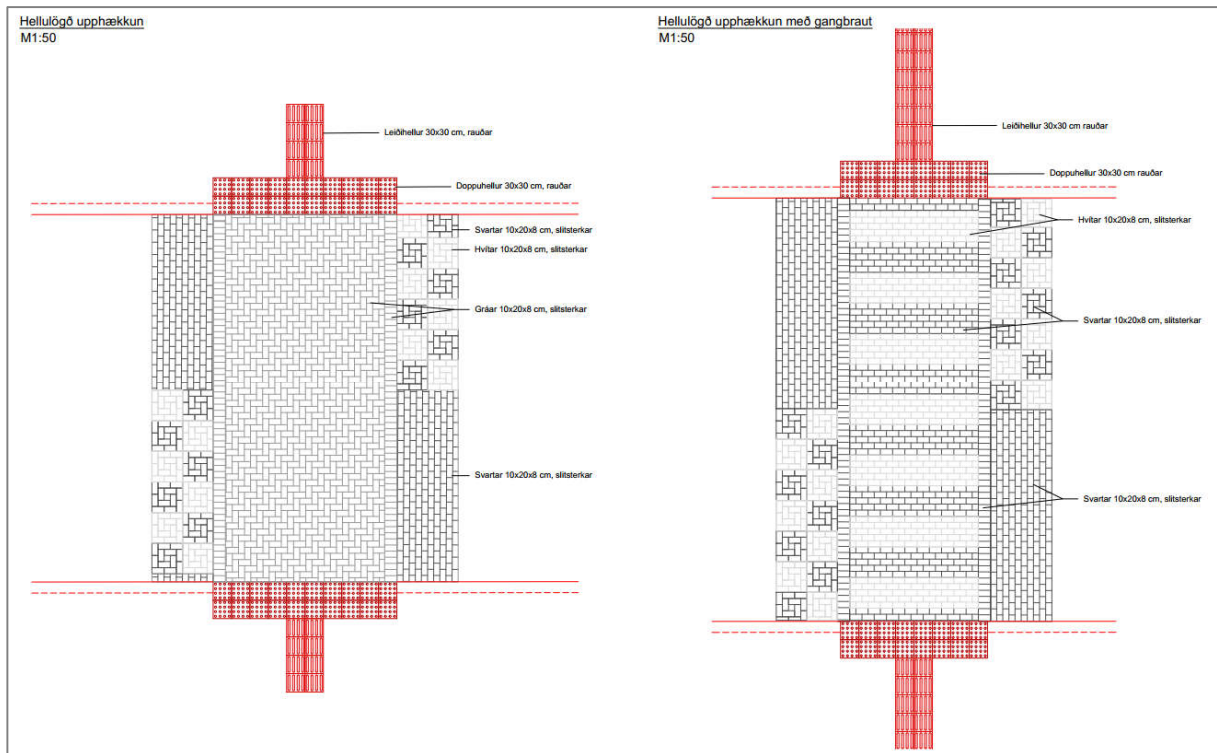
MYND 9 Hellulagðar upphækkanir, til hægri með gangbrautarmörkingum.
