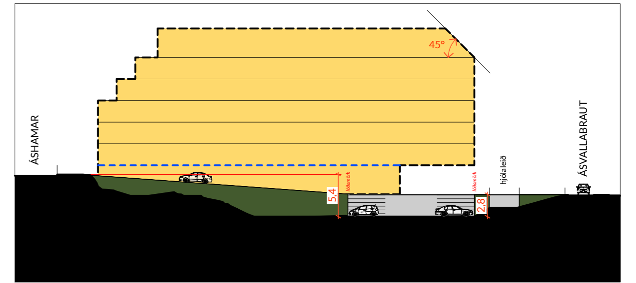
Snið CC 1:500
