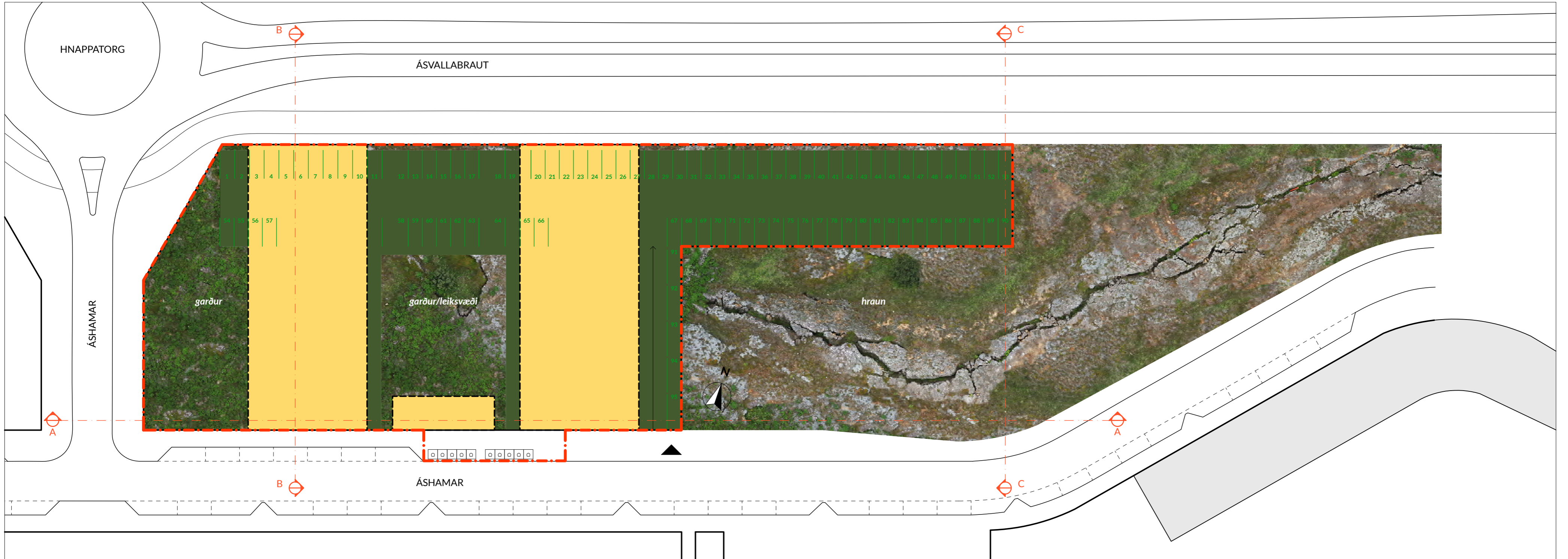
Lóðaskipulag 1:500
