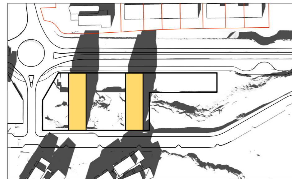
Skuggar - Vor/Haust - 20/03 13:30
